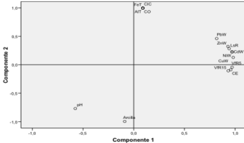
Figura 2. Análisis de componentes principales entre propiedades de un suelo andisol y un vertisol
