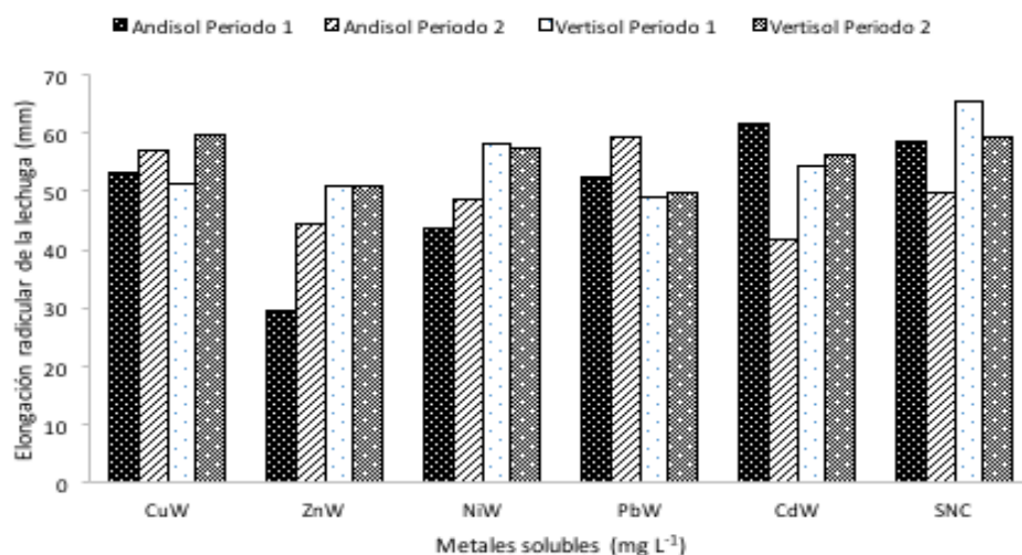
Figura 1. Elongación radicular de la lechuga (mm) en los diferentes tratamientos. SNC: Suelo no contaminado; S.D: Desviación estándar; *: Diferencias significativas en relación con el SNC ( p < 0,05 )
